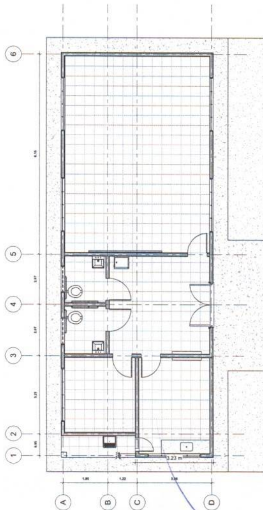
02. EIXOS (TERREO) 1:50
