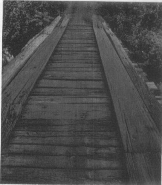
Imagem 03 – ponte de madeira com desgaste por falta de manutenção na passa roda, transversinas, pilares.
