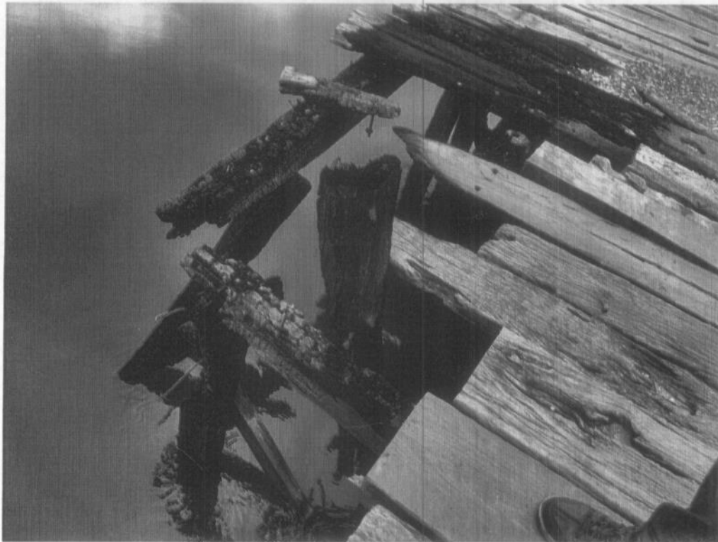
Imagem 05 – pilares, transversinas e pranchas queimados.
