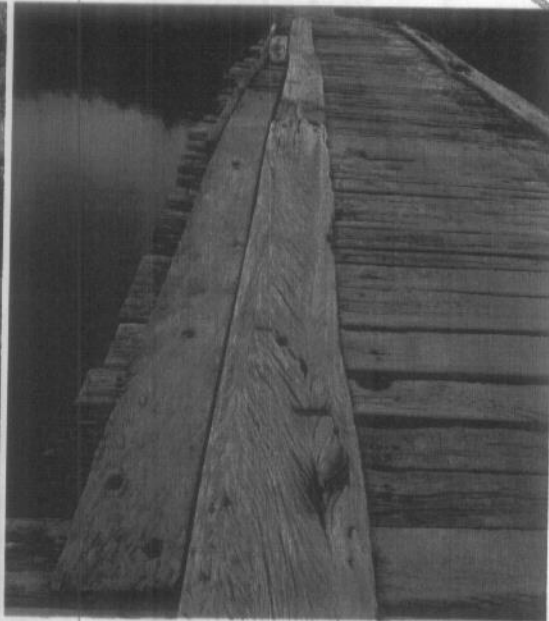
Imagem 03 – ponte de madeira com desgaste por falta de manutenção na passa roda, transversinas, pilares.
