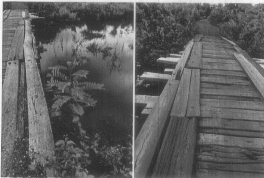
Imagem 02 – ponte de madeira com desgaste por falta de manutenção na passa roda, transversinas, pilares.
