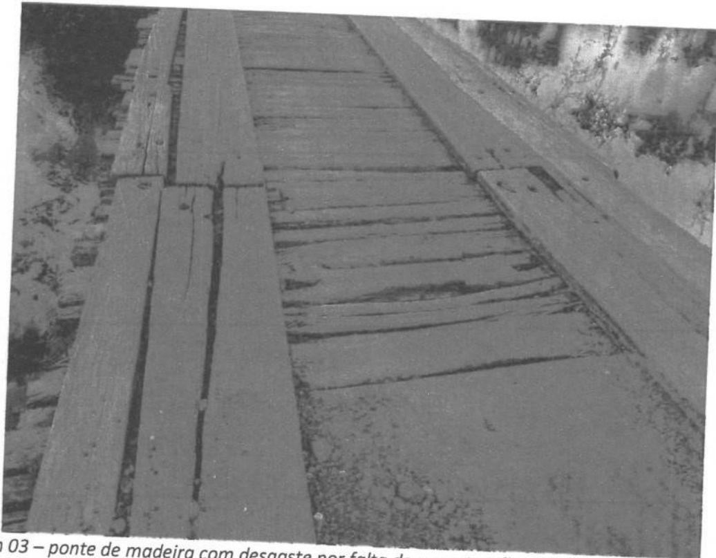
Imagem 03 – ponte de madeira com desgaste por falta de manutenção na passa roda, transversinas, pilares.
