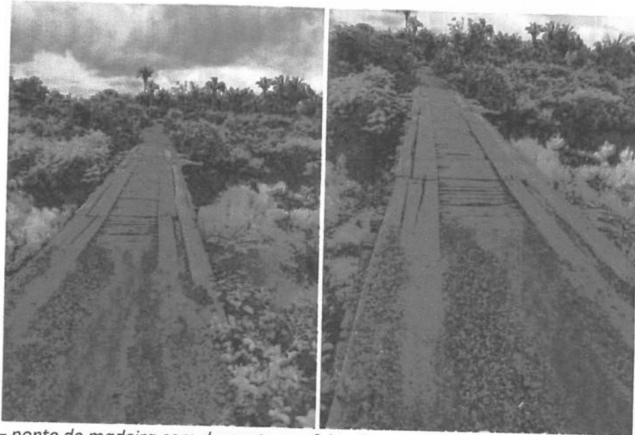
Imagem 01 – ponte de madeira com desgaste por falta de manutenção na passa roda, transversinas, pilares.
