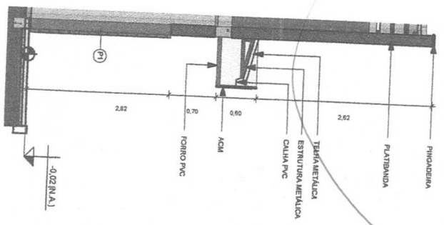
2 DETALHE DA FACHADA 1 : 50
