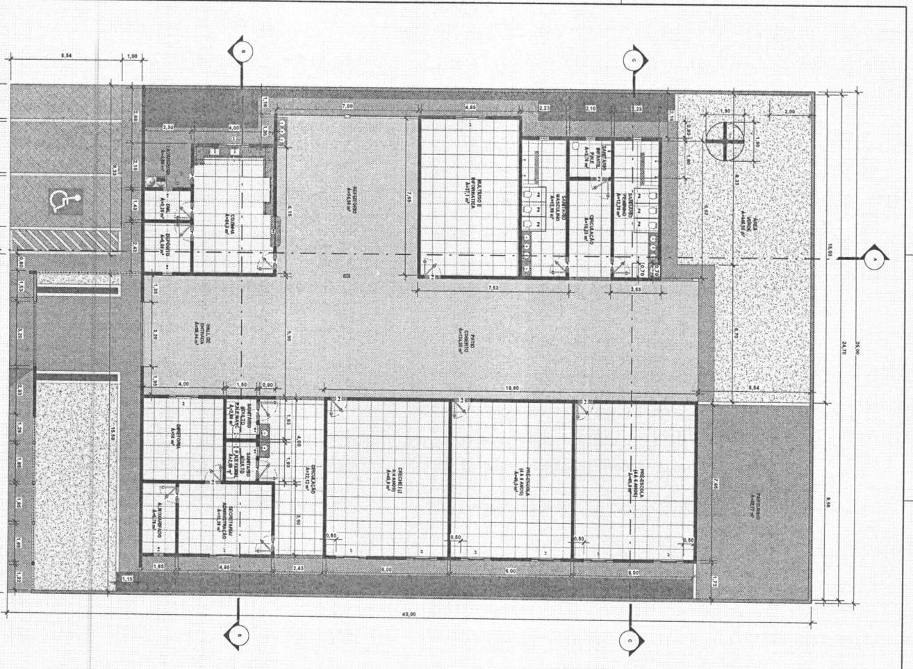
1 1 - 1/25 PLANTA BAIXA
