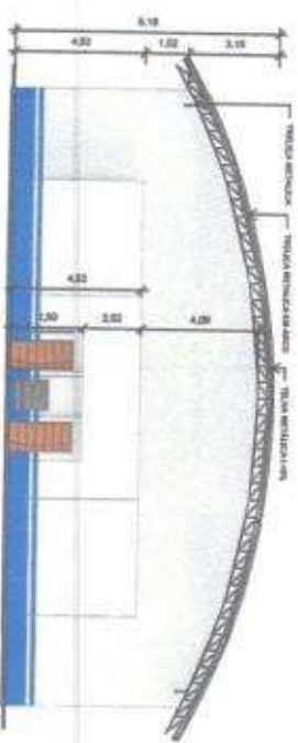
4 CORTE DD 1:100
