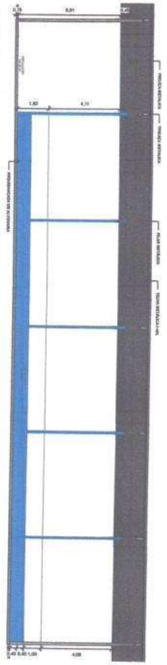
1 CORTE AA 1:75
