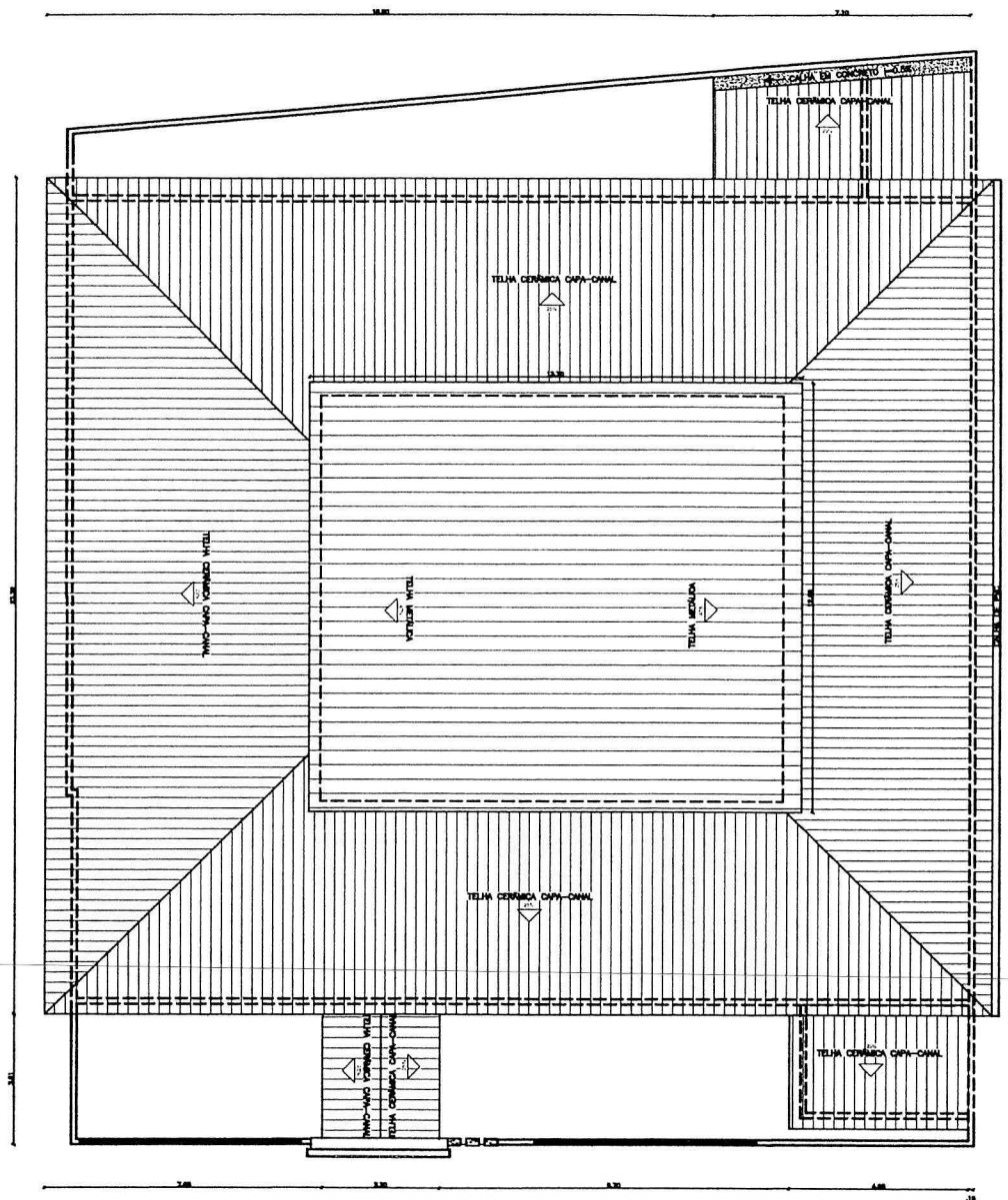
PLANTA DE COBERTURA esc 1:75
