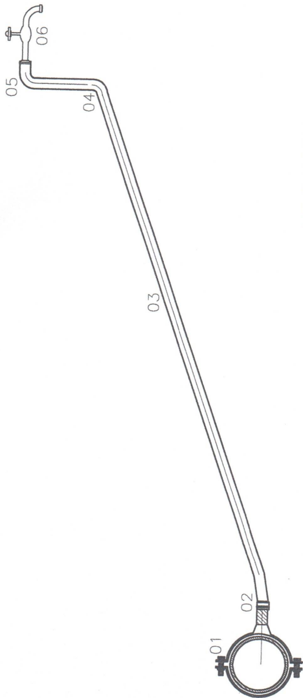
LIG. DOMICILIAR ESCALA 1:25
