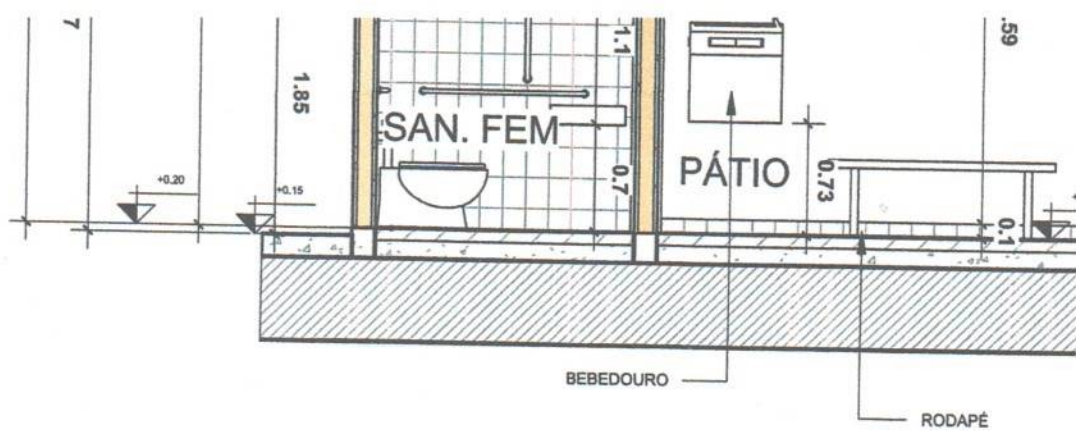
2 CORTE B-B 1:50
