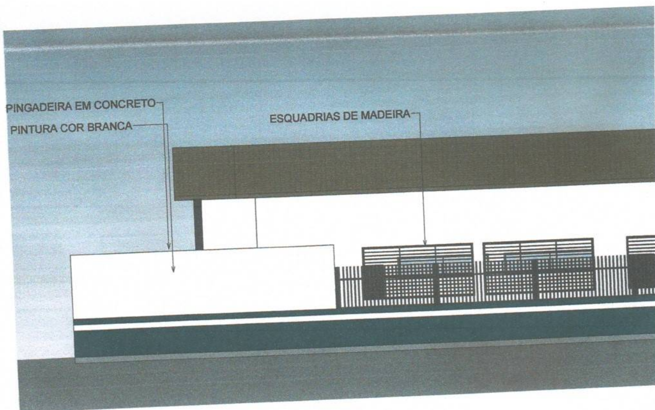
1 FACHADA LESTE ESCALA 1:100
