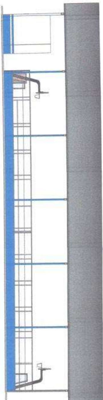
1 FACHADA NORTE 1 : 75
