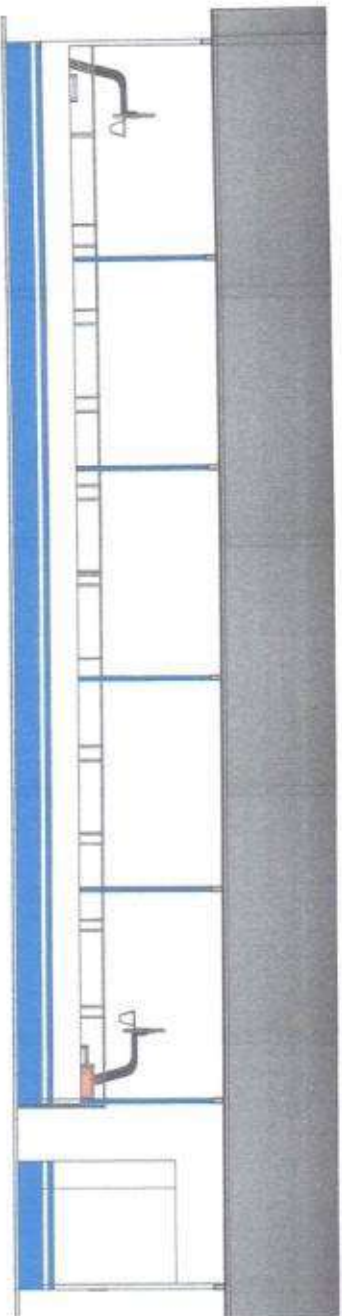
2 FACHADA SUL 1 : 75
