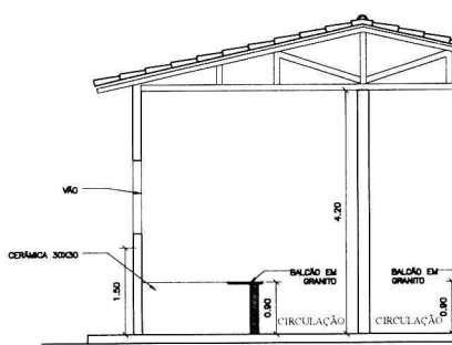
● CORTE BB ESC.: 1/100
