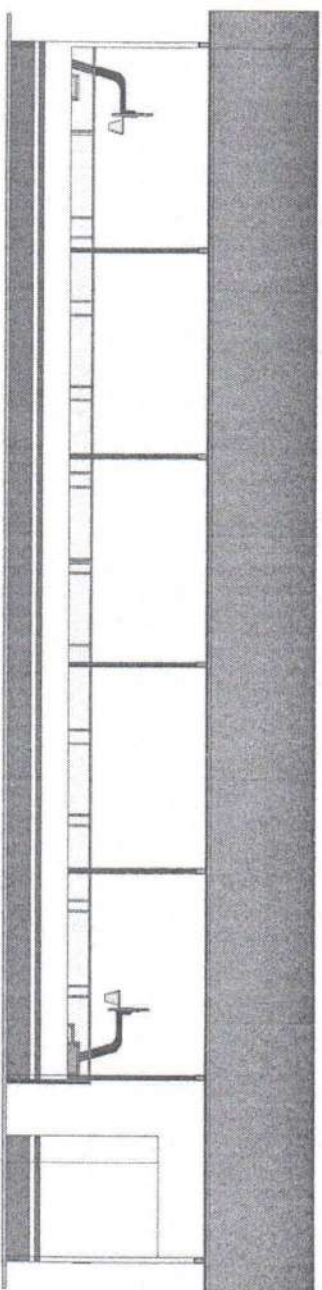
2 FACHADA SUL 1 : 75
