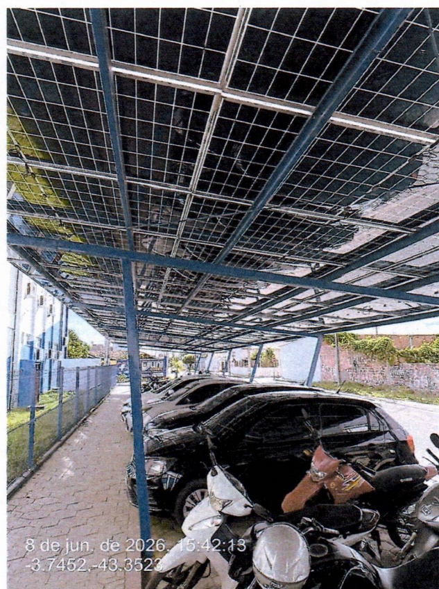
Imagem 05 – Estrutura metálica de estacionamento
