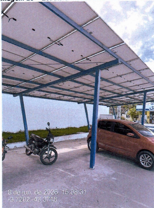
Imagem 24 – Estrutura metálica de estacionamentos
